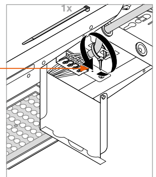
Vormontierte Klemme zur Zugentlastung des Stromkabels über einfachen Kabelclip (nicht im Lieferumfang enthalten)
