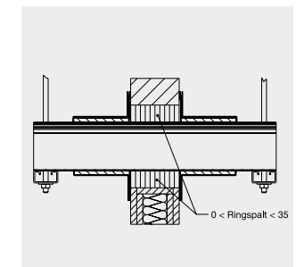
Kanal durchgängig Wandöffnung \geq Kanalquerschnitt
