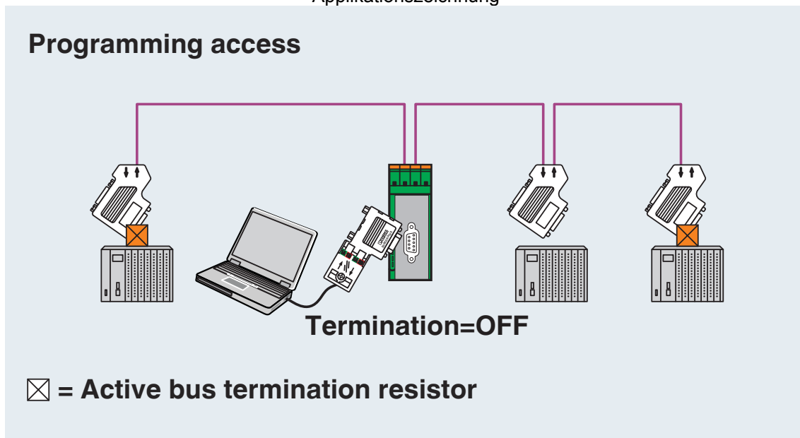
Feste Serviceschnittstelle im (Profi-)Bussystem
