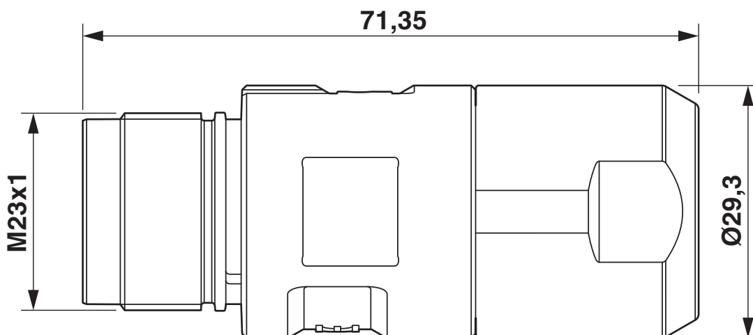
Maßzeichnung
