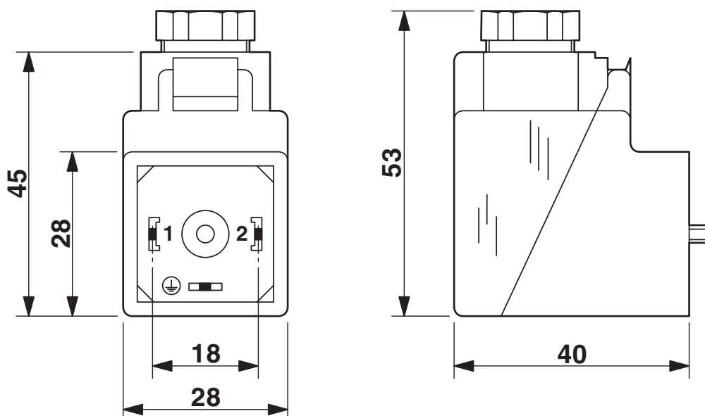
Maßzeichnung
