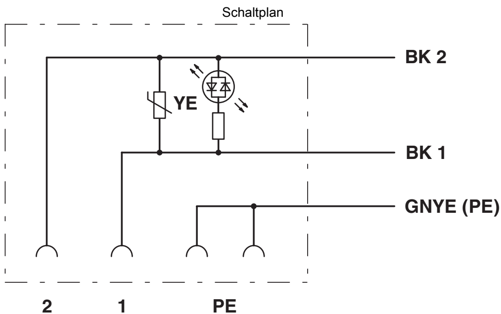
Polbild Ventilstecker, Bauform A
