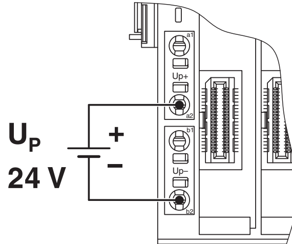
Anschlusszeichnung
