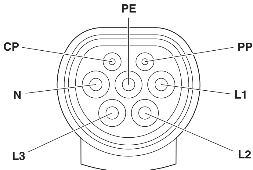
Schemazeichnung
