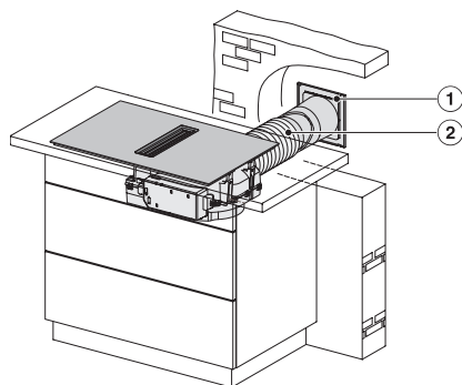
KMDA7676FL, KMDA7876FL – Einbauvariante 11 Abluft – Skizze
