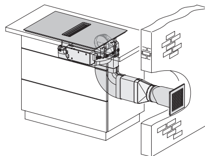
KMDA7676FL, KMDA7876FL – Einbauvariante 10 Abluft – Skizze
