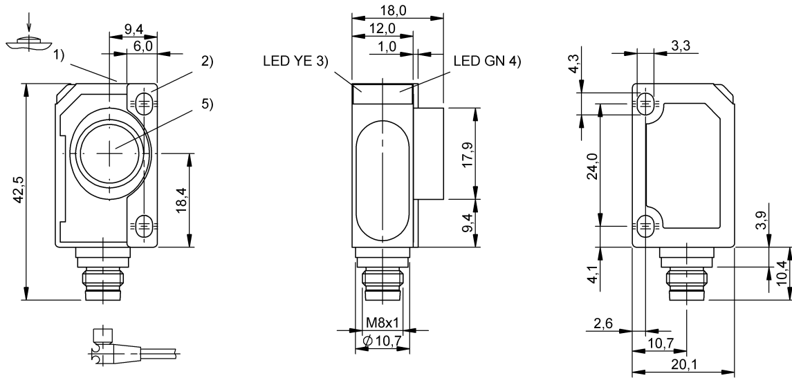
1) Sensor einstellen, 2) Befestigungsplatte, 3) Zustandsanzeige, 4) Betriebsspg./Betriebsart, 5) Achse Ultraschallwandler
