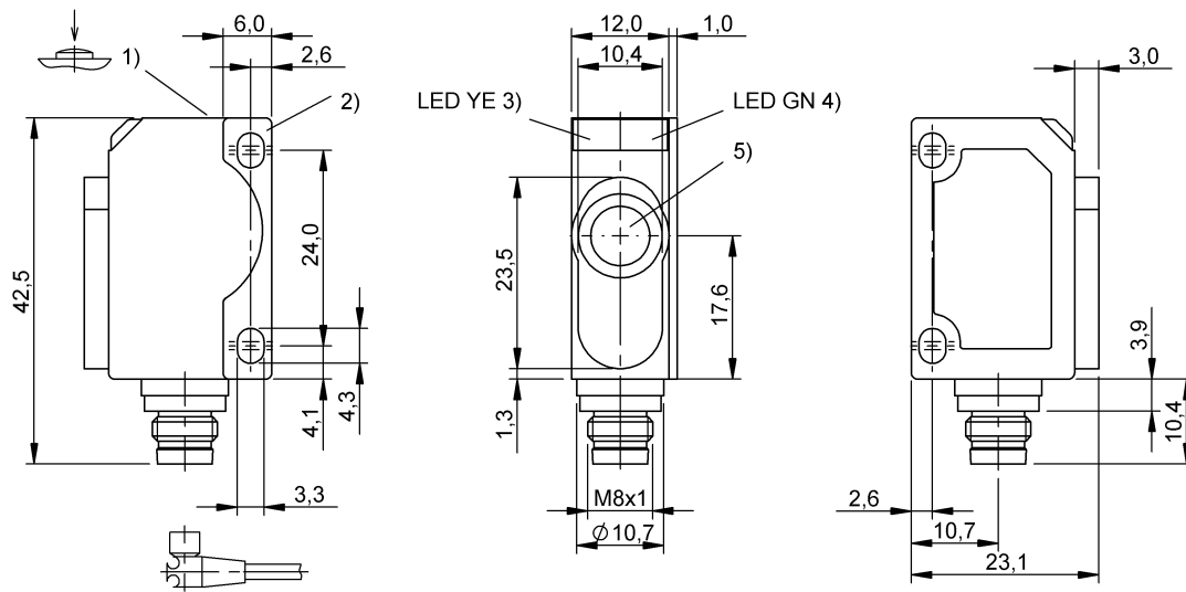
1) Sensor einstellen, 2) Befestigungsplatte, 3) Zustandsanzeige, 4) Betriebsspg./Betriebsart, 5) Achse Ultraschallwandler
