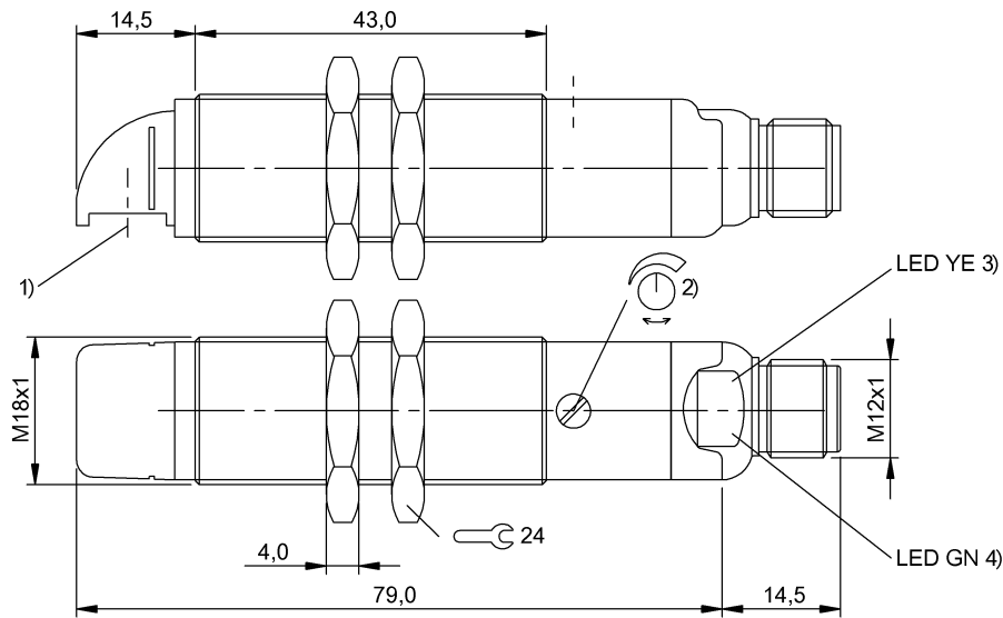
1) Optische Achse, 2) Sn, 3) Ausgangsfunktion, 4) Betriebsspannung
