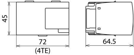
Maßbild DV MOD TNC 255
