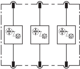
Prinzipschaltbild DV MOD TNC 255
