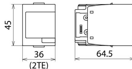
Maßbild DV MOD TN 255
