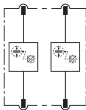
Prinzipialschaltbild DV MOD TN 255
