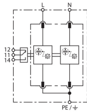
Principalschaltbild DV M2 TN 255 FM
