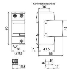
Maßbild DV M2 TN 255 FM
