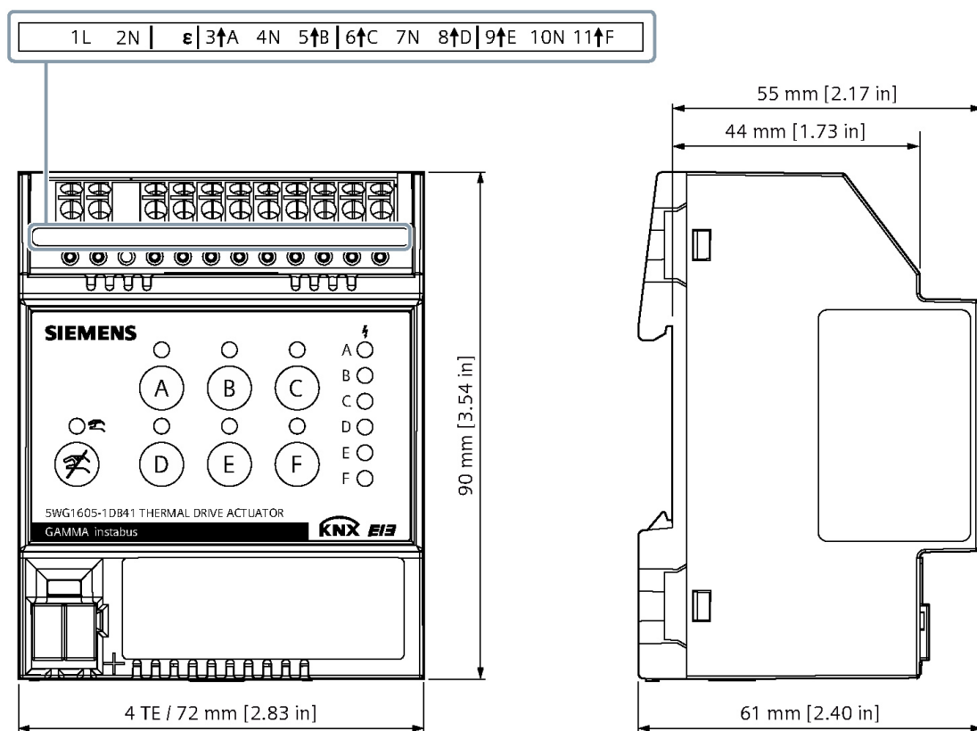
Abb. 15: Thermoantriebsaktor N 605D41, 6 x AC 24...230 V
