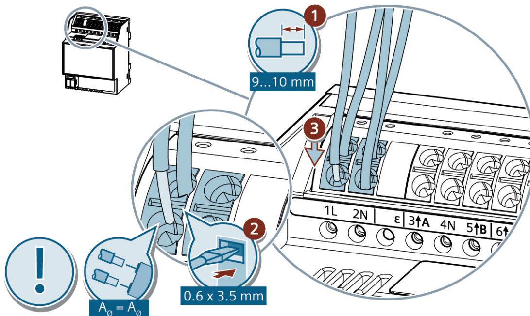
Abb. 9: Thermoantriebsaktor N 605D41, 6 x AC 24...230 V
