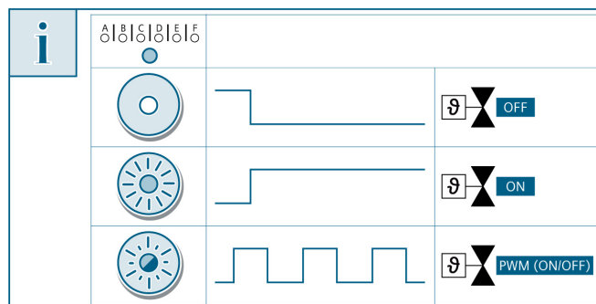
Abb. 12: Thermoantriebsaktor N 605D41, 6 x AC 24...230 V
