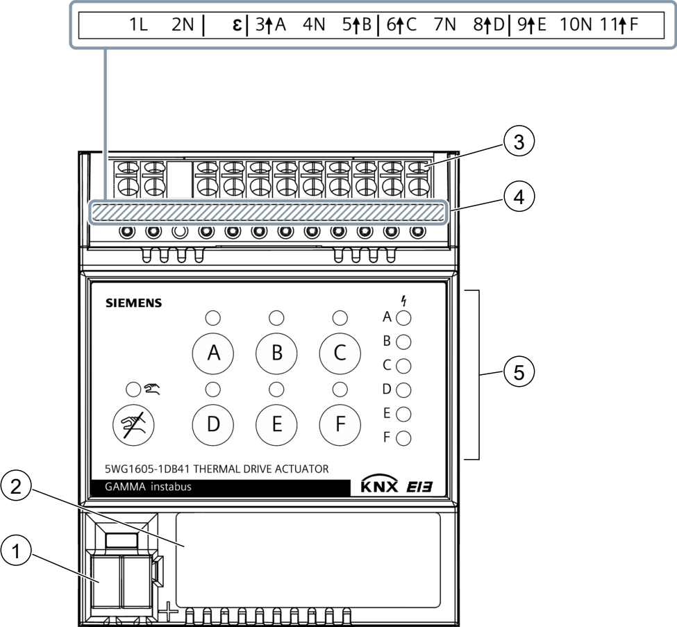
Abb. 7: Lage und Funktion der Anschlüsse und Beschriftung, Thermoantriebsaktor N 605D41, 6 x AC 24...230 V
