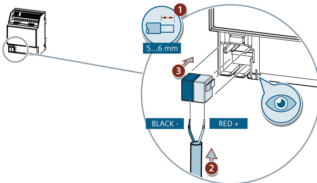
Abb. 10: Thermoantriebaktor N 605D41, 6 x AC 24...230 V
