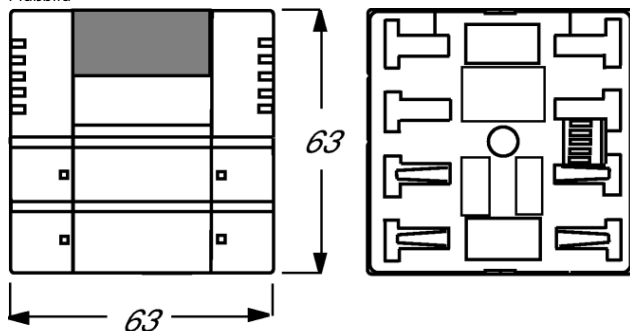
Maßbild
