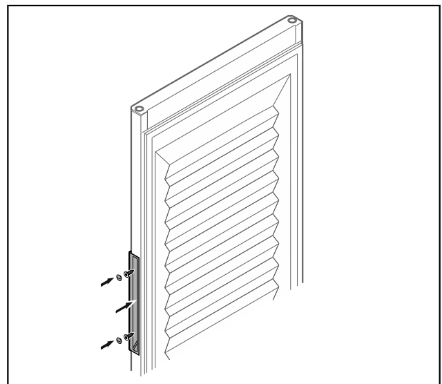
Fig. 26 Geschäumte Tür*
