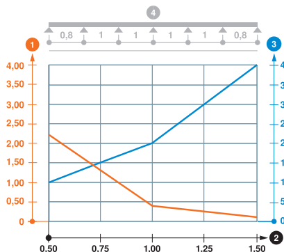
Belastungsdiagramm Kabelrinne Typ MKR 15 100 FS
