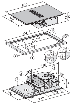
KMDA7272FL, KMDA7473FL – flächenbündig – Skizze
