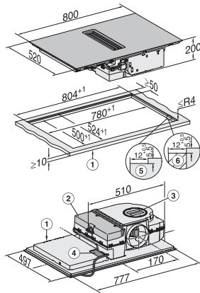
KMDA7272FL, KMDA7473FL – flächenbündig – Skizze
