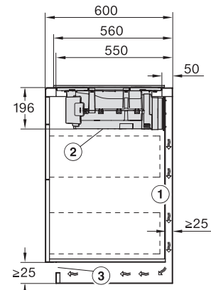
KMDA7272FL, KMDA7473FL – Skizze Seitenansicht aufliegend, Plug&Play
