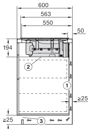
KMDA7272FR, KMDA7473FR – Skizze Seitenansicht aufliegend, Plug&Play
