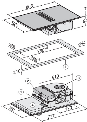
KMDA7272FR, KMDA7473FR – aufliegend – Skizze
