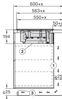
KMDA7272FR, KMDA7473FR – Skizze Seitenansicht aufliegend+X, Plug&Play
