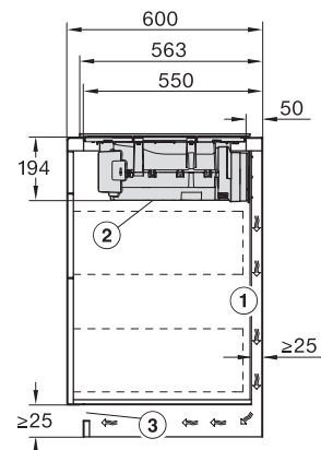
KMDA7272FR, KMDA7473FR – Skizze Seitenansicht aufliegend, Plug&Play
