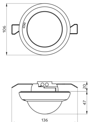
Bemaßung 93516
