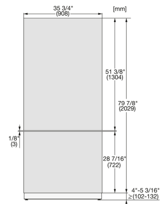
KFP3615ed/cs, KFP3625ed/cs, KFP3614ed/cs, KFP3624ed/cs Frontplatte, Frontmaße, MasterCool
