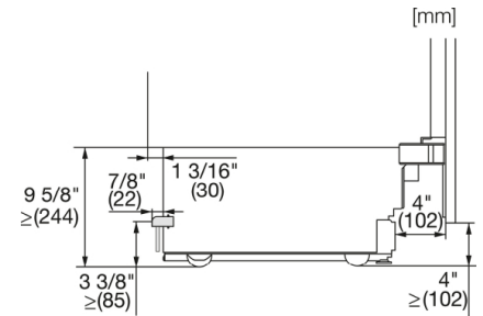
KF2901Vi/SF, KF2911Vi/SF, KF2801Vi/SF, KF2811Vi/SF, KF2981Vi/SF, Seitenansicht, MasterCool, Skizze
