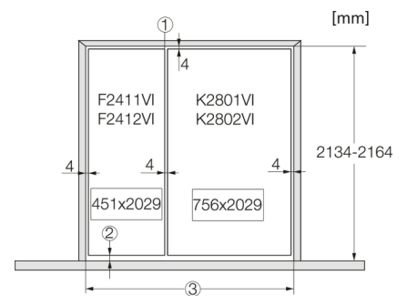
Bemaßungsbeispiel Side-by-side-Kombination MasterCool (Skizze) *Fußnote (nur für EUROPA)
