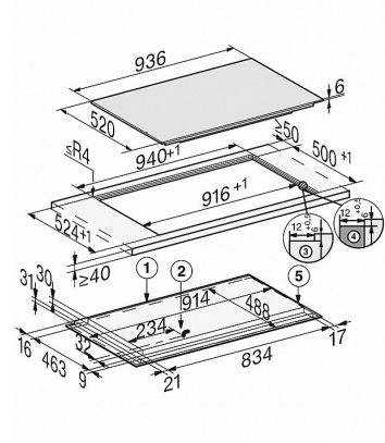
KM 7999 FL (Skizze) - flächenbündig
