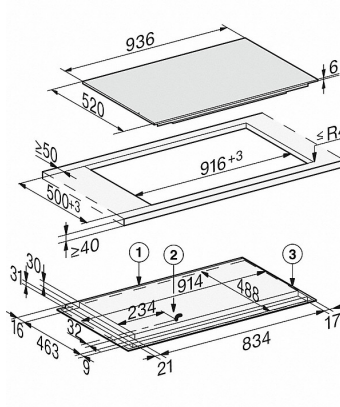
KM 7999 FL (Skizze) - aufliegend
