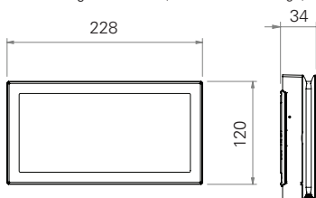
Maßangaben in mm (Wandaufbaumontage)
