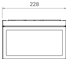
Maßangaben in mm (Deckenaufbaumontage)
