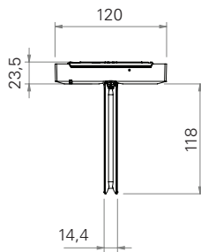
Maßangaben in mm (Wandaufbaumontage)
