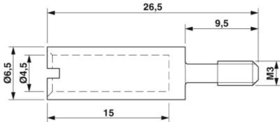
Maßzeichnung
