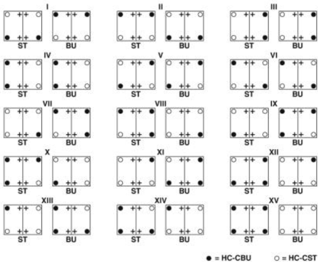
Schemazeichnung
