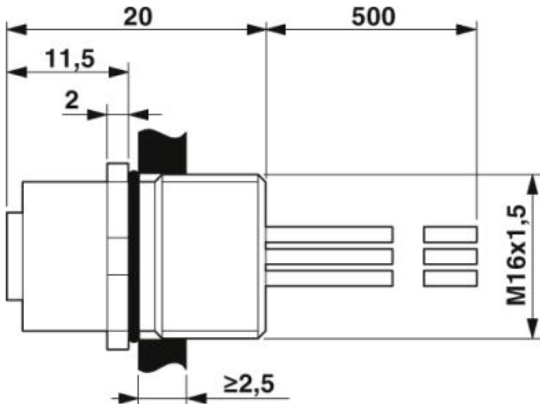
Maßzeichnung
