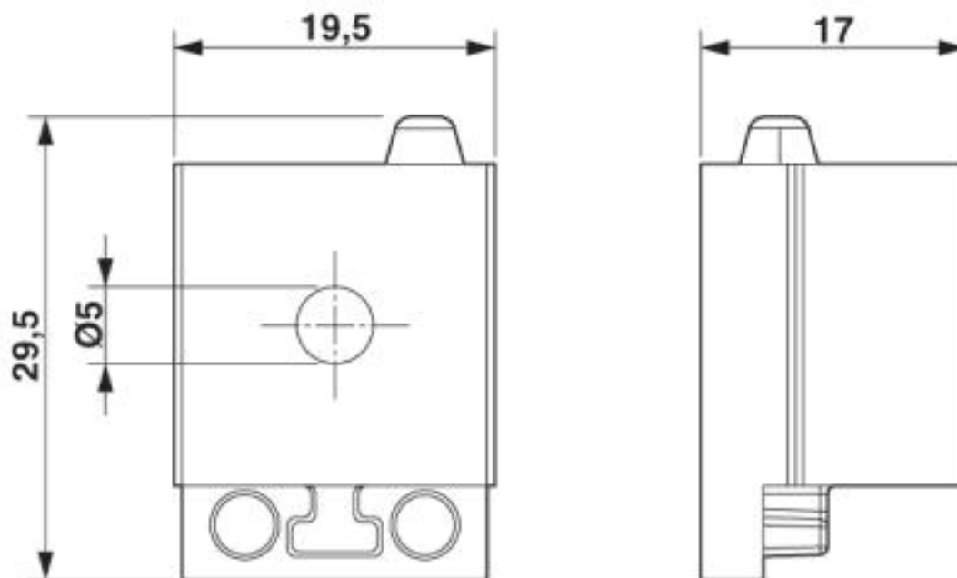
Maßzeichnung
