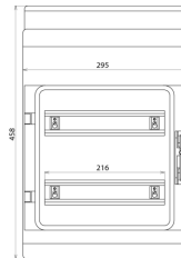
Maßbild IGA 24 IP54
