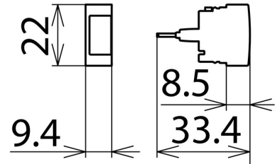
Maßbild EM 2 DRL
