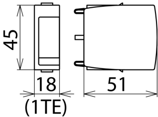
Maßbild DG MOD 150
