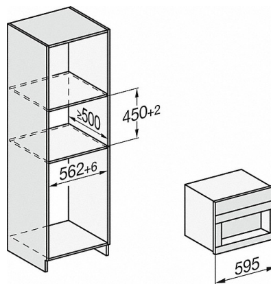
CVA7000 (Einbauskizze)
