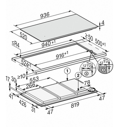
KM 7697 FL, KM 7897 FL (Skizze) flächenbündig
