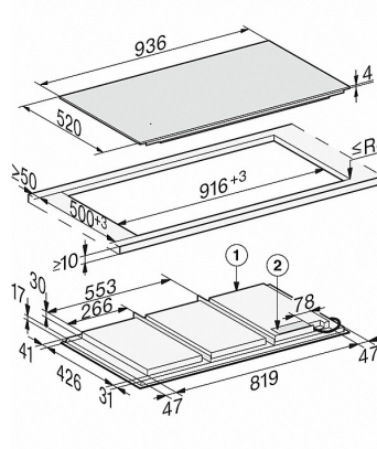
KM 7697 FL, KM 7897 FL (Skizze) aufliegend
