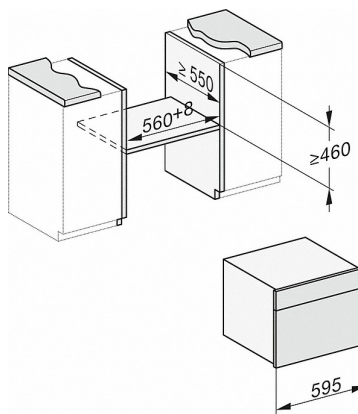
DG7x4x, DGM7x4x, DGC7x4x, DGC7x4xX Skizze
