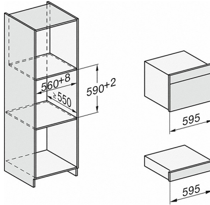
ESW7x10, Skizze
