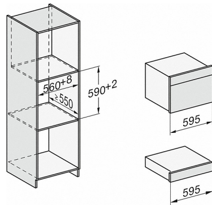
ESW7x10, Skizze
