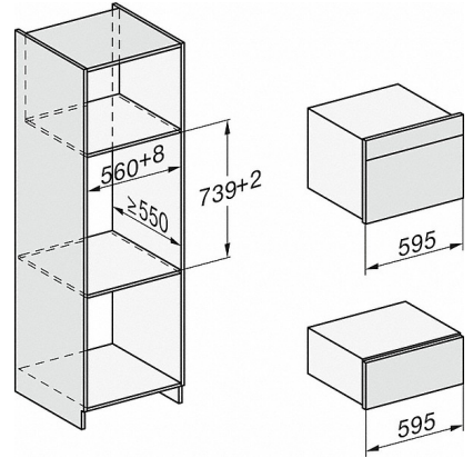
ESW7x20, Skizze
