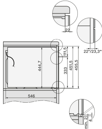
H7x40BM/BMX, Skizze, Unterbau
