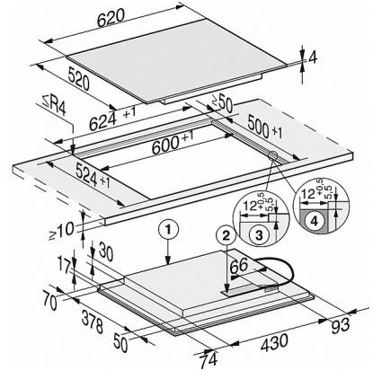
KM 6329, KM 7564 flächenbündig (Skizze)
