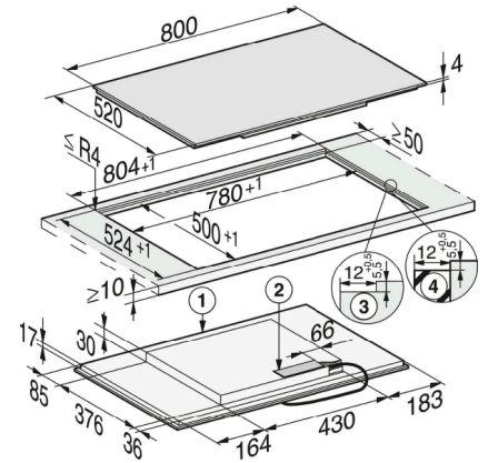
KM 7474 FL flächenbündiger Einbau (Skizze)
