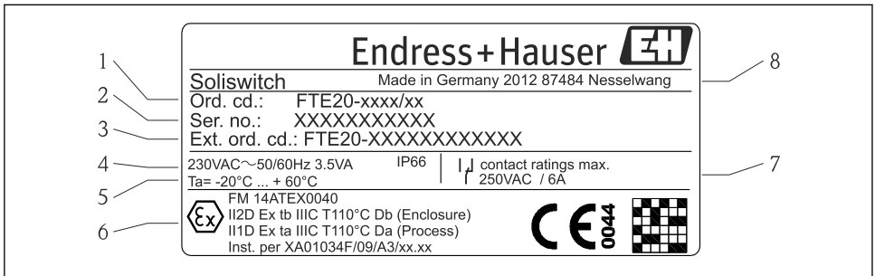
1 Typenschild des Soliswitch FTE20 (beispielhaft)
