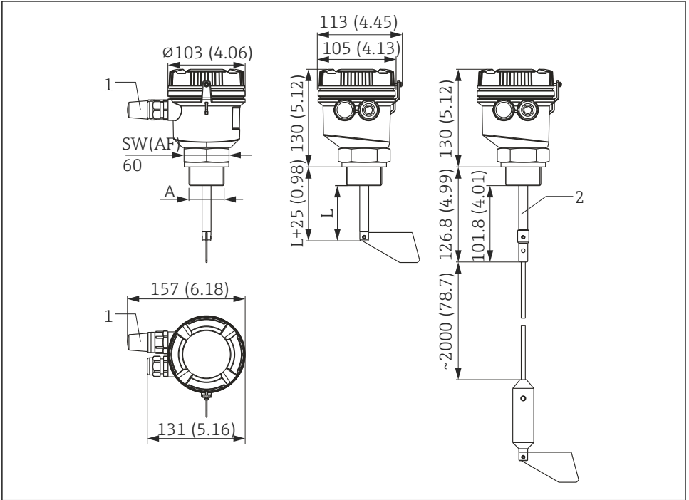
16 Abmessungen des Füllstandgrenzschalters, Angaben in mm (in)
