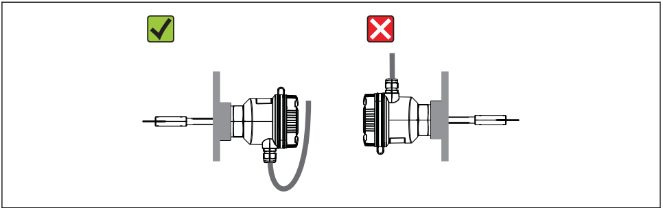
5 Richtige Position des Gehäuses
