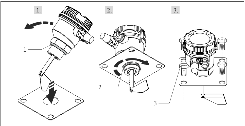
6 Montage der Flanschversion
