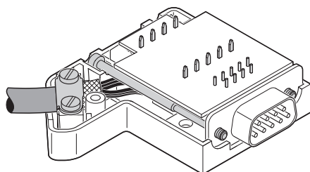
Rechtsseitige Kabelzuführung
