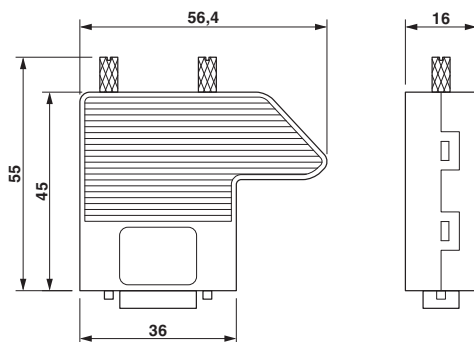
Maßzeichnung
