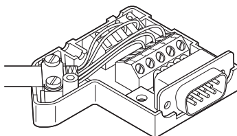
Schemazeichnung
