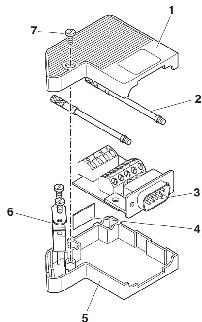
Explosions-Zeichnung
