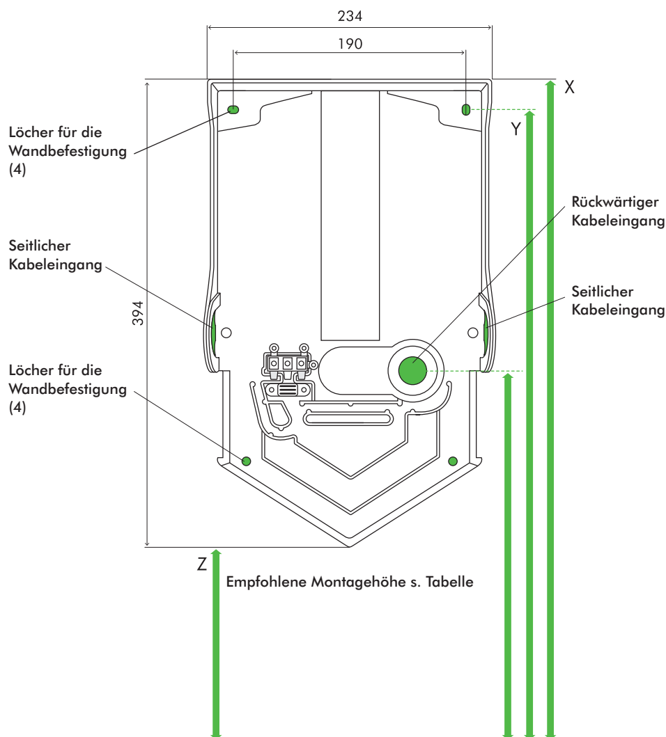
RÜCKANSICHT
