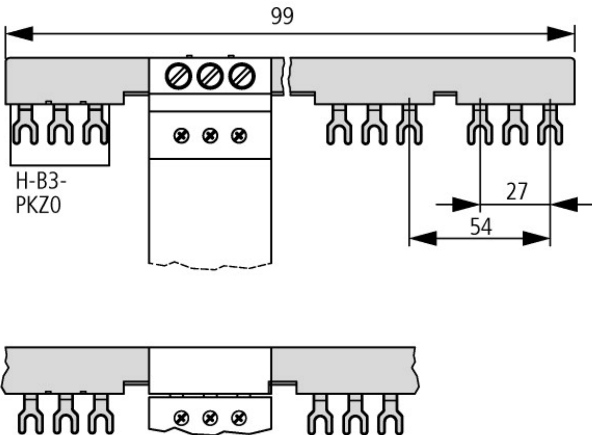
Drehstromschienenblock
