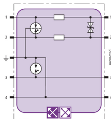
Principalschaltbild BXT ML2 BD S 12
