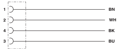
Kontaktbelegung des M12-Stecker und der M12-Buchse
