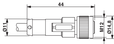
Buchse M12 x 1, gerade
