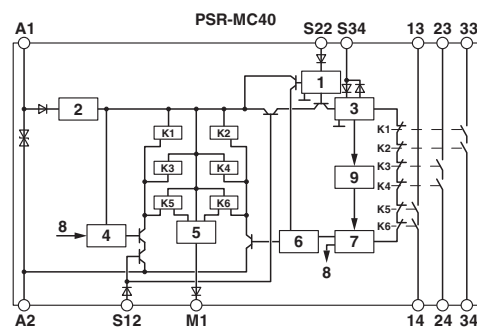
Blockschaltbild
