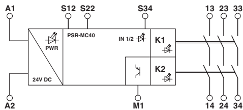
Blockschaltbild
