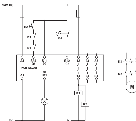
Schaltplan
